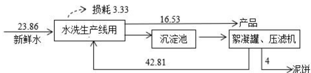
图 2-2 本次技改项目水平衡图，单位： \text{m}^3/\text{d}
