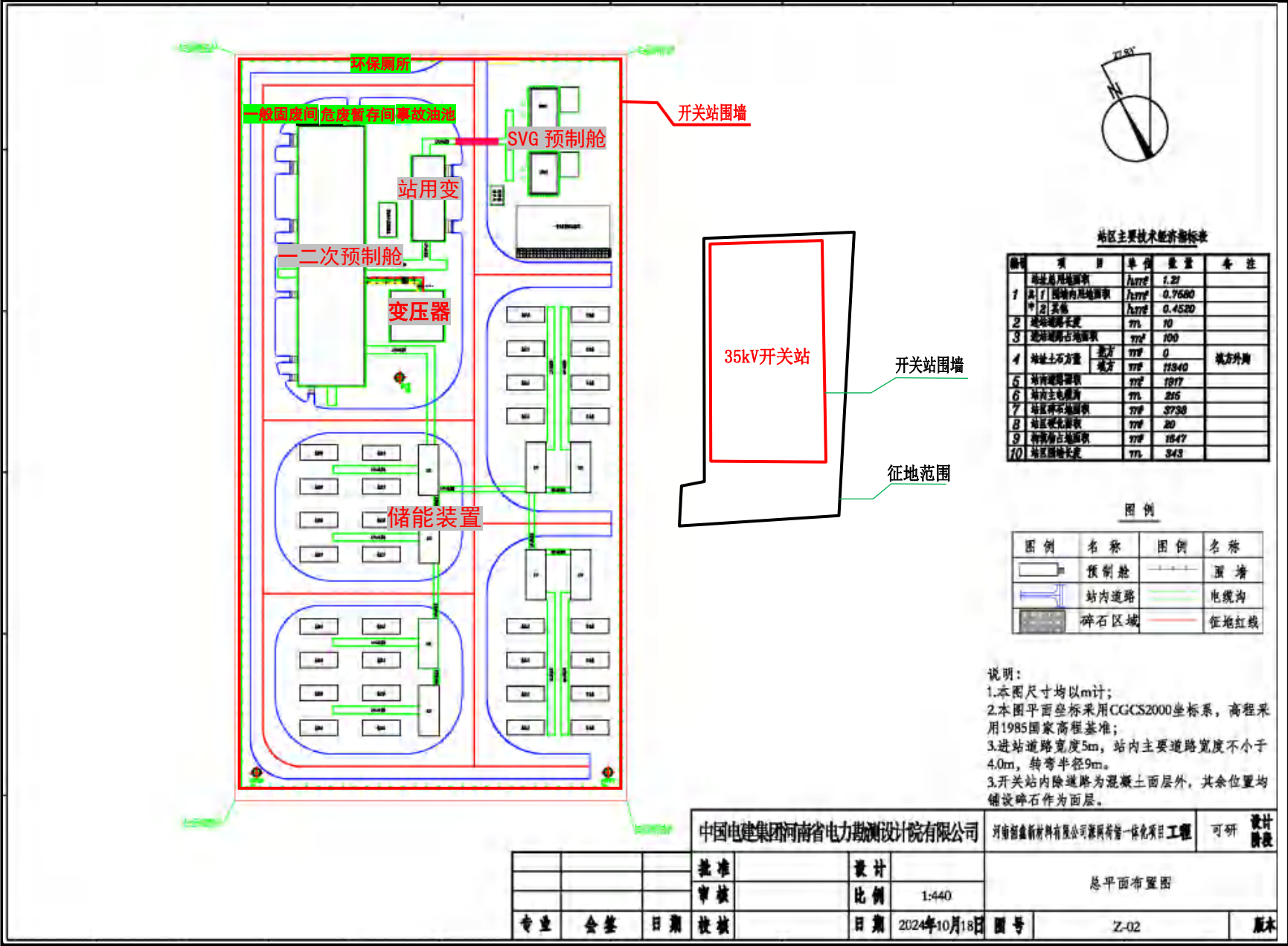
附图 3-2 新建 35kV 开关站平面布置及环境保护措施分布示意图
