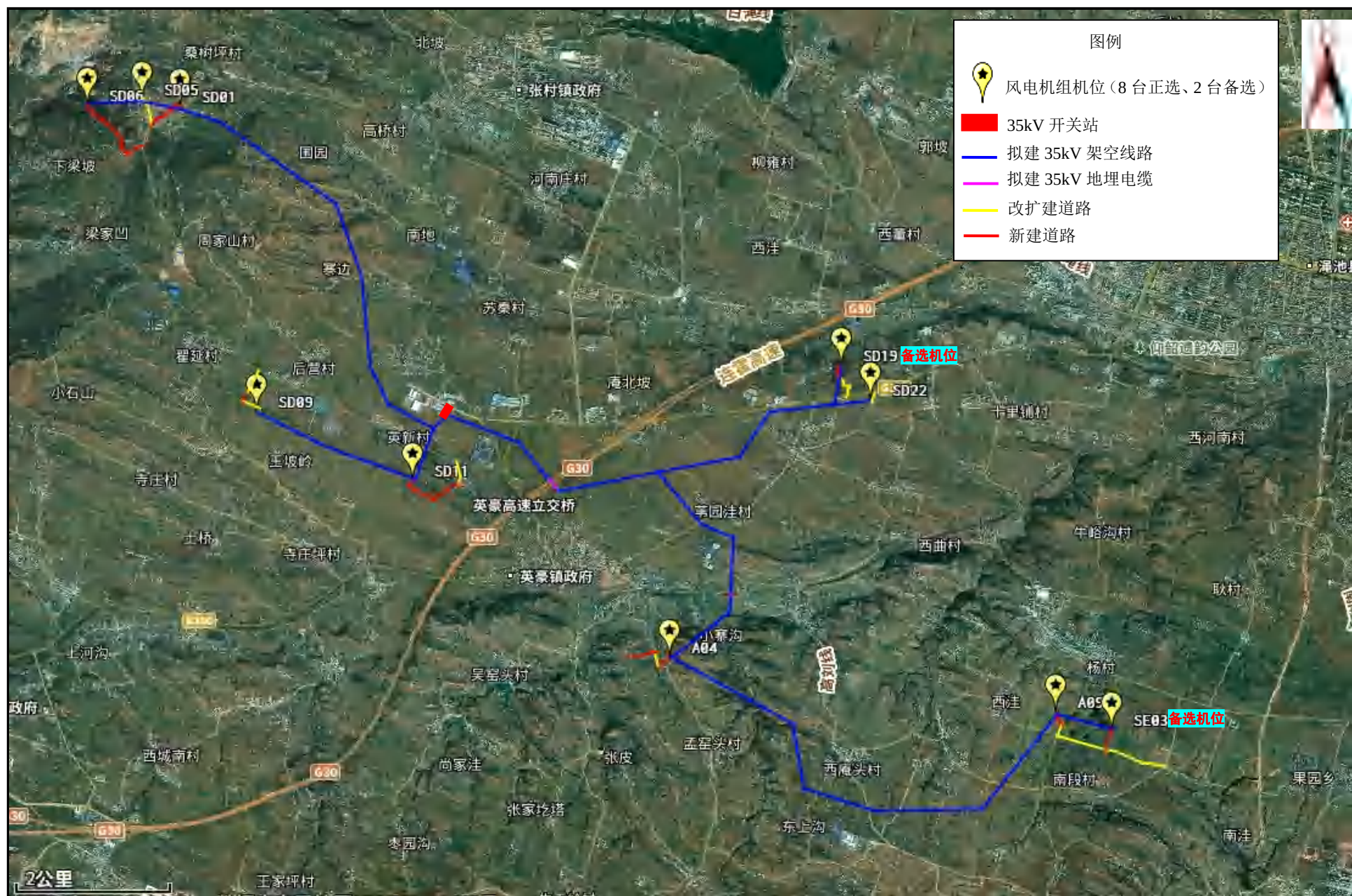
附图 3-1 项目总平面布置示意图
