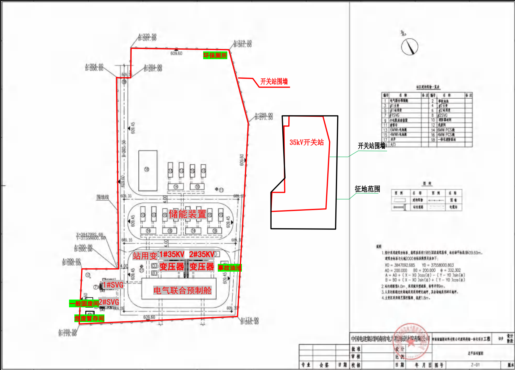
附图 3-3 新建 35kV 开关站平面布置及环境保护措施分布示意图
