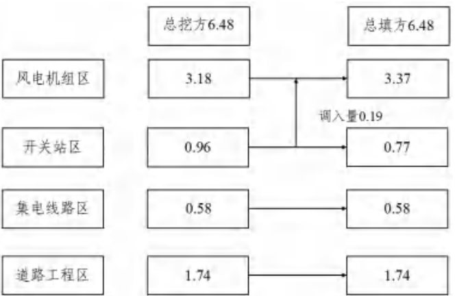
图2-1 土石方平衡流向图 单位: 万m 3
