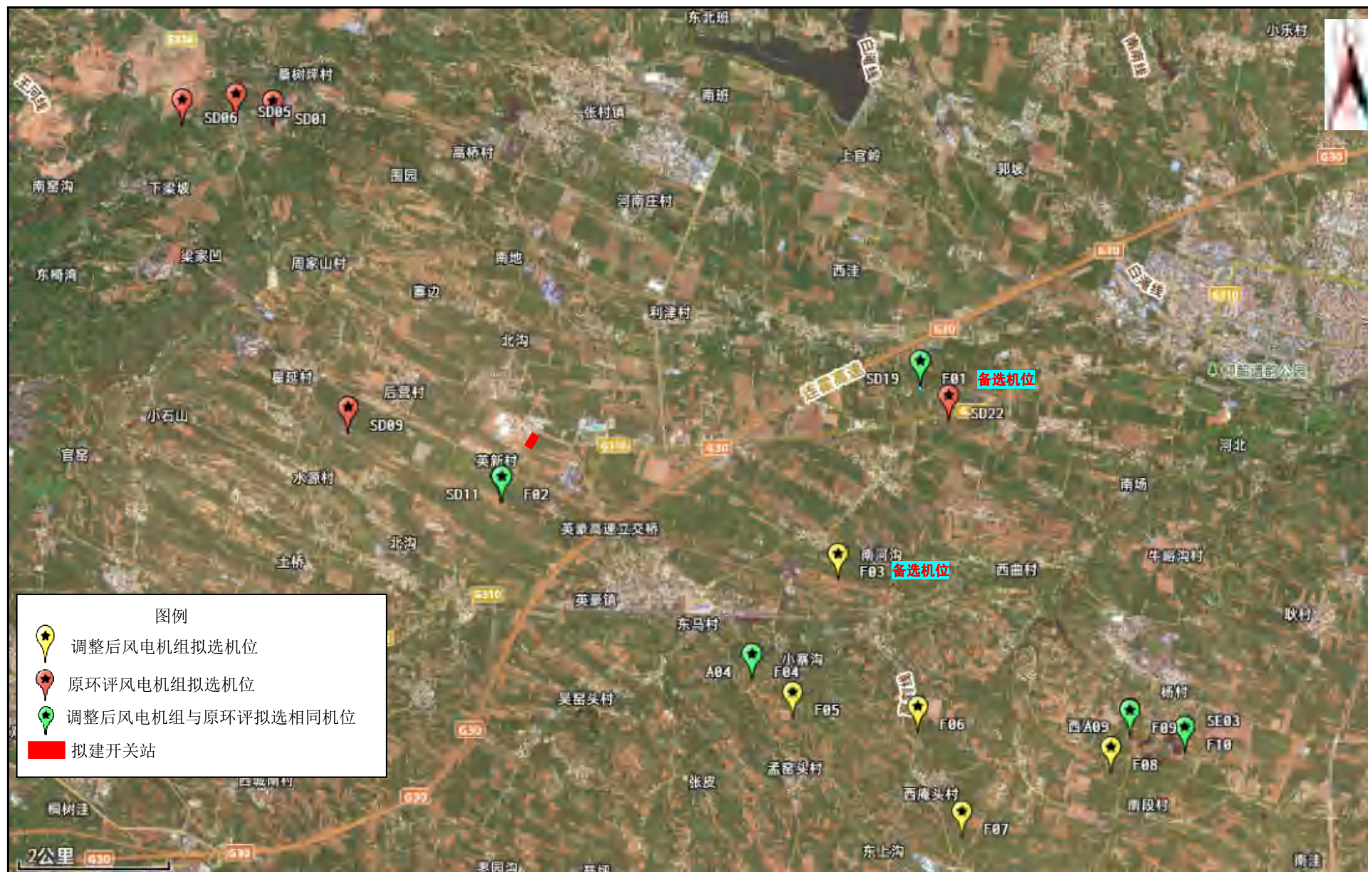
附图 3-2 项目原环评阶段与现阶段风机布置对比示意图
