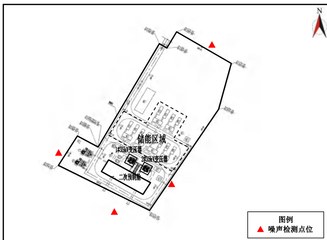
图5-1 运营期开关站环境检测布点示意图
