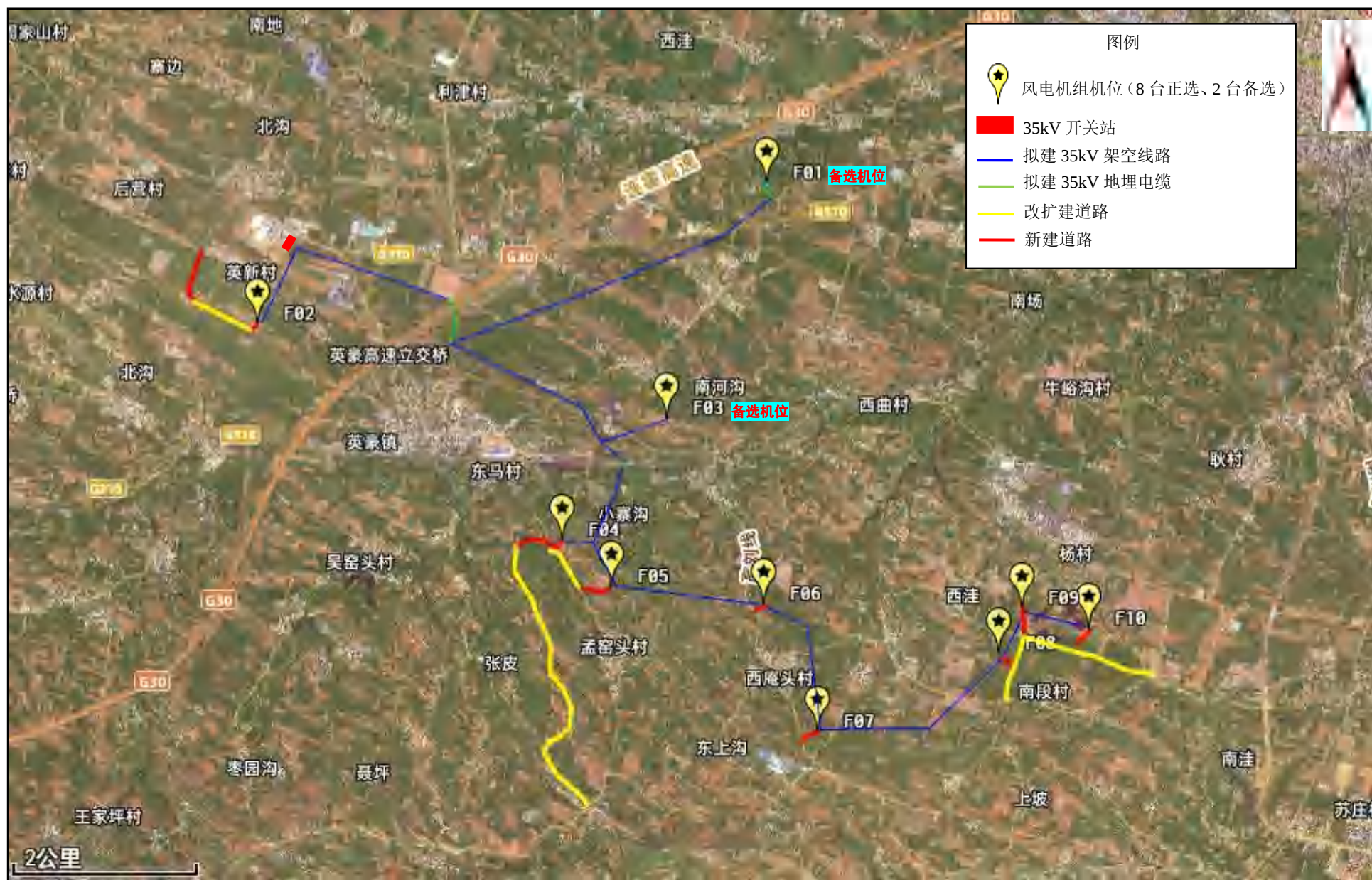
附图 3-1 项目总平面布置示意图
