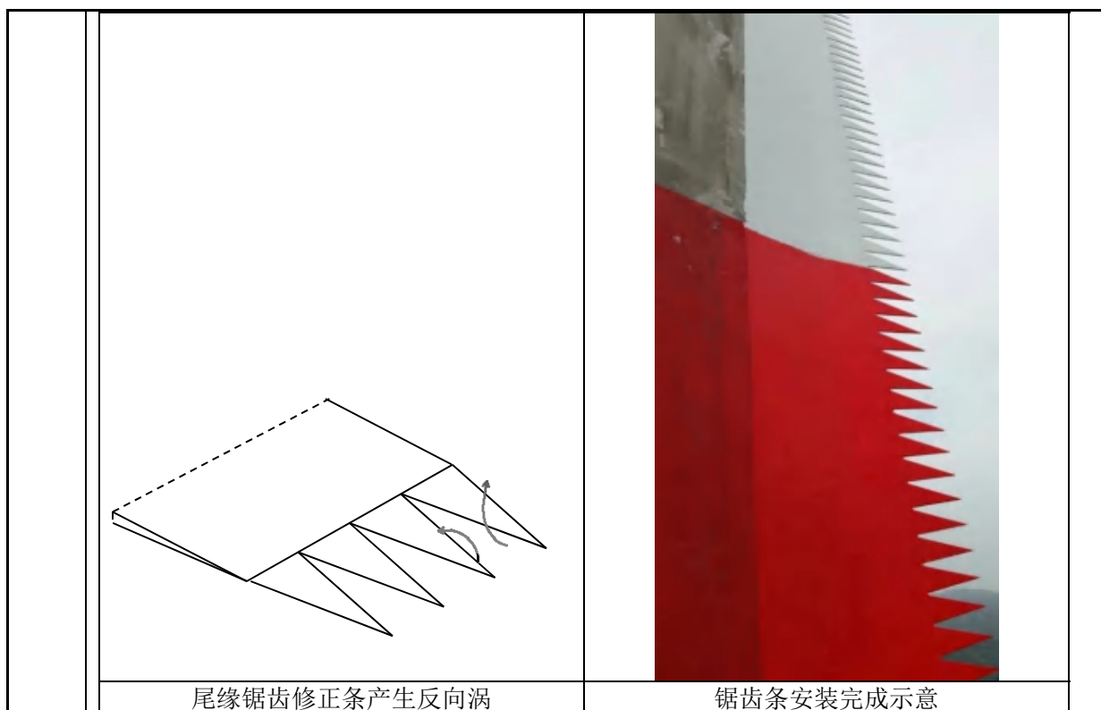
图 4-3 风机尾缘锯齿条示意图
