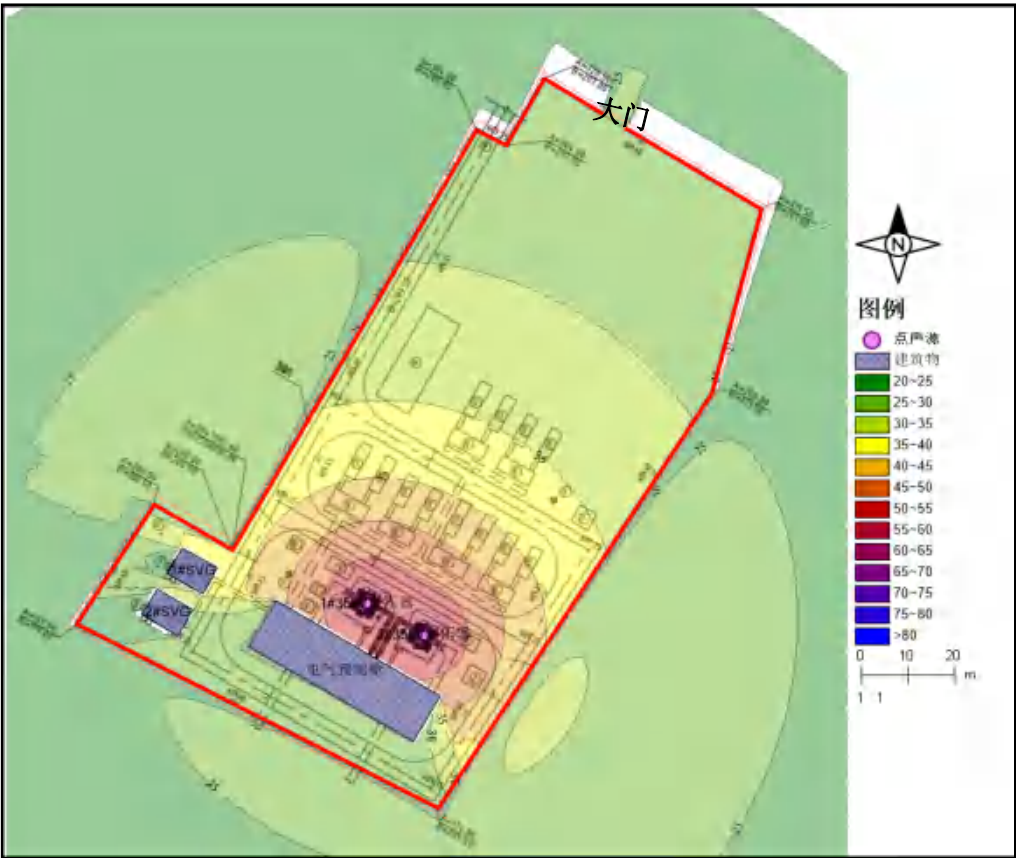
图 4-5 运营期噪声贡献值预测结果
