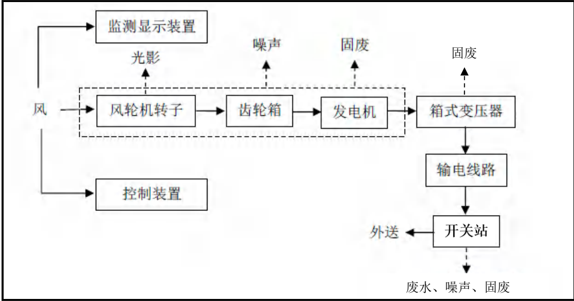
图4-2 运营期工艺流程及产污环节示意图
