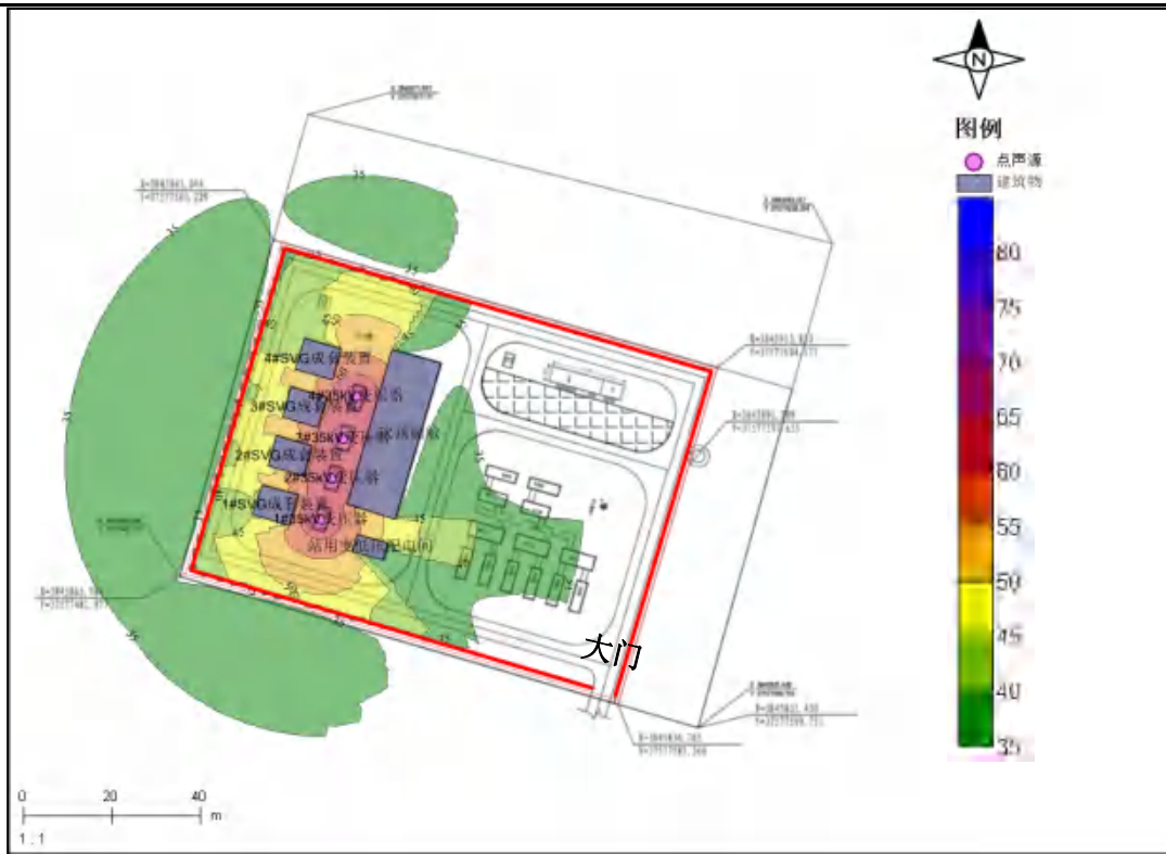
图 4-5 运营期噪声贡献值预测结果
