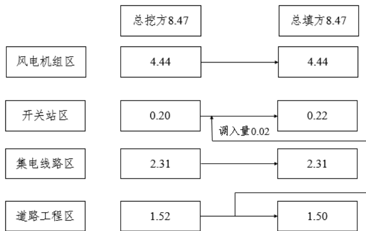
图2-1 土石方平衡流向图 单位: 万m 3
