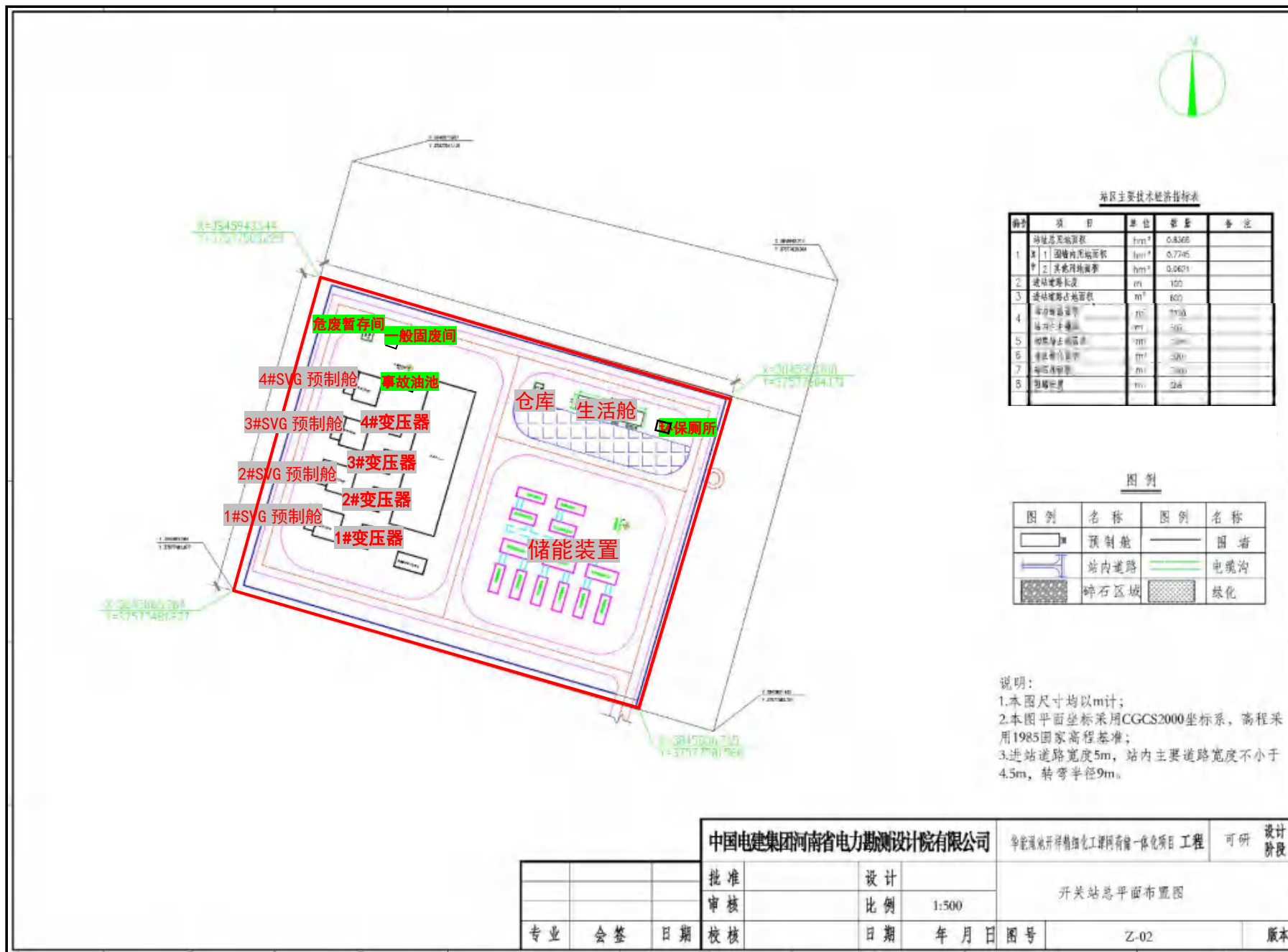
附图 3-3 新建 35kV 开关站平面布置及环境保护措施分布示意图
