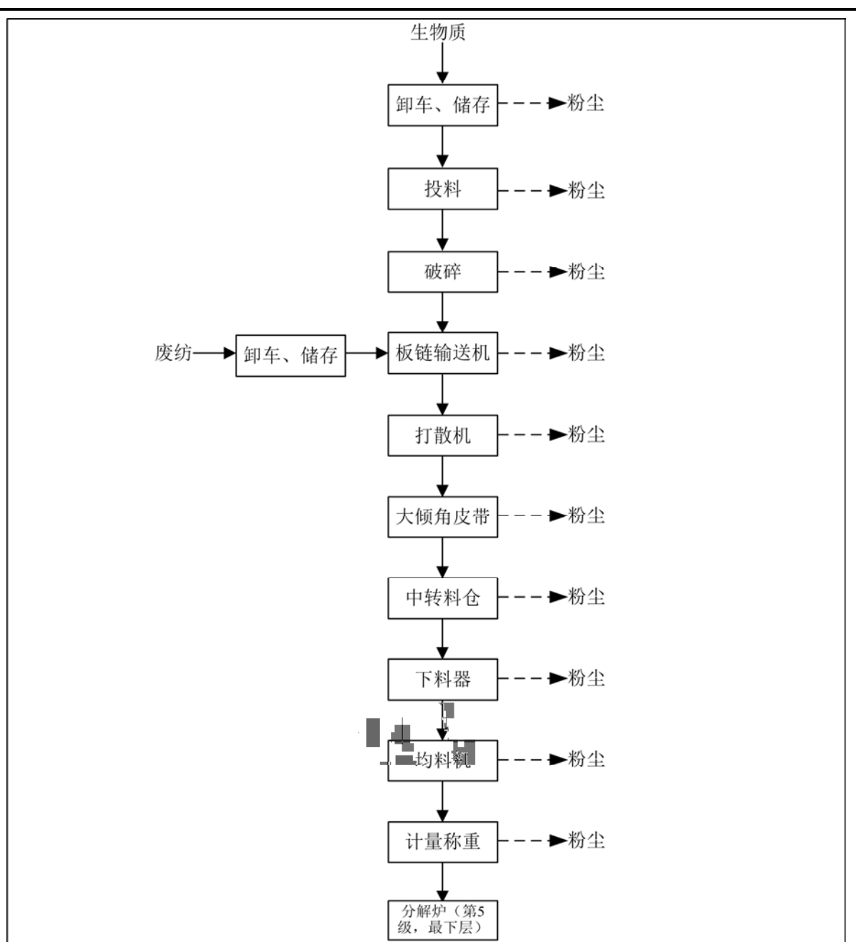
图 2-5 本次工程（替代燃料储存车间）工艺流程及产污环节示意图
