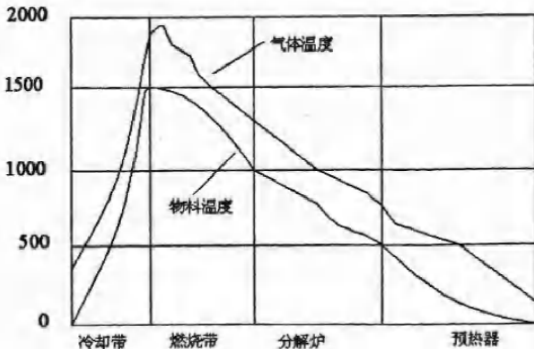
图 2-2 物料与气体的温度 (°C) 分布图
