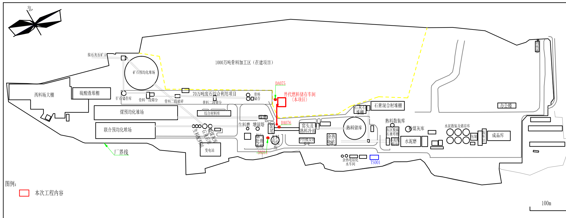
附图3 厂区总平面布置图
