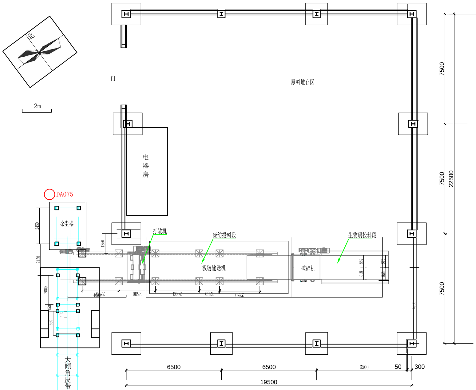
附图4 替代燃料储存车间设备布局图
