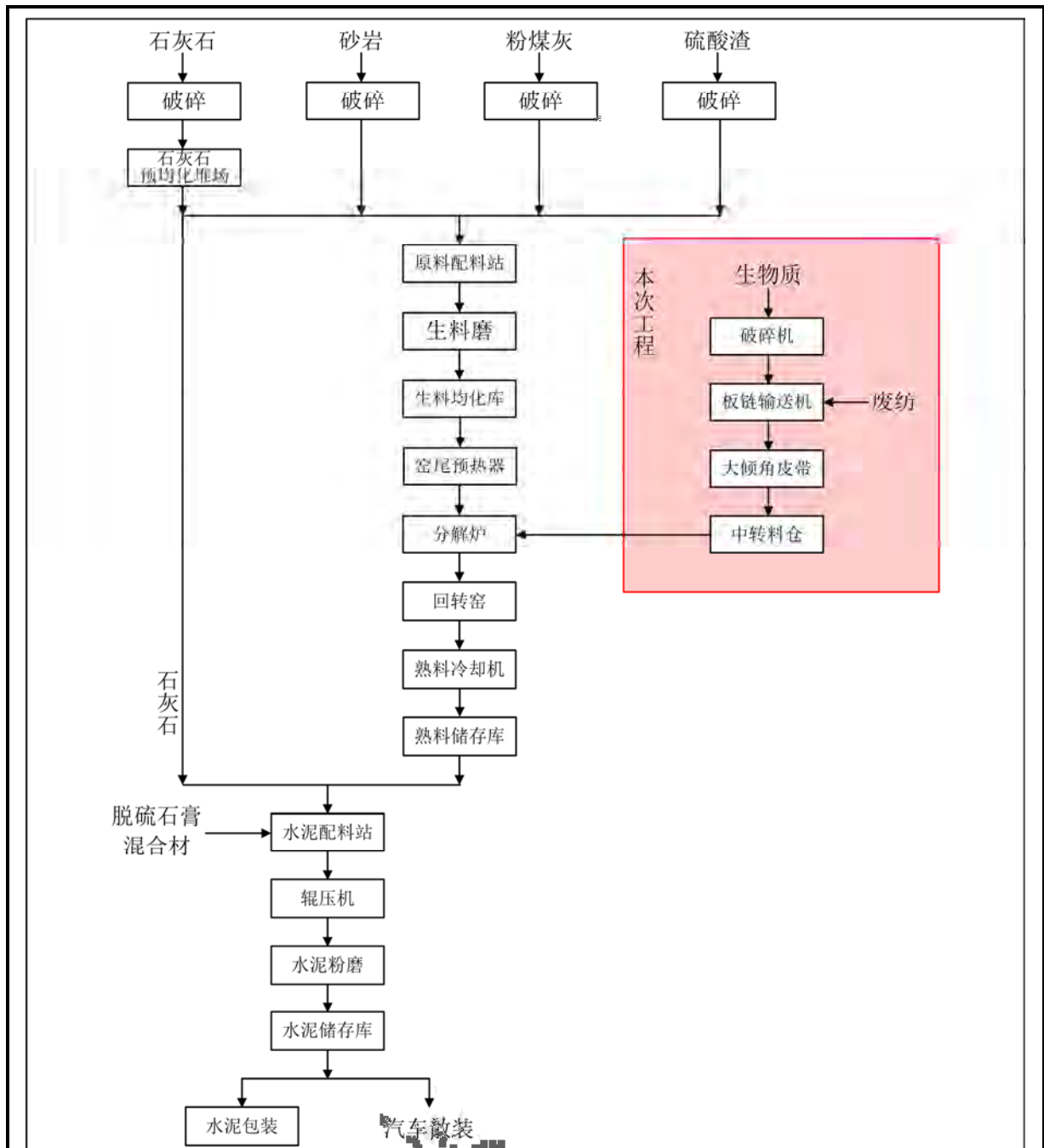
水泥生产整体生产工艺流程图
